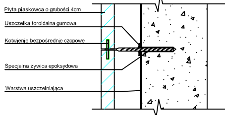
KOTWIENIE BEZPOŚREDNIE DO ŚCIANY BETONOWEJ
