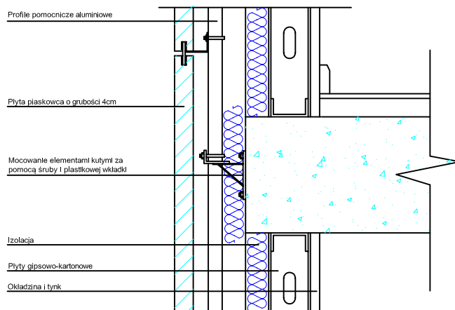
KONSTRUKCJA POMOCNICZA MIĘDZY ELEMENTAMI KUTYMI
