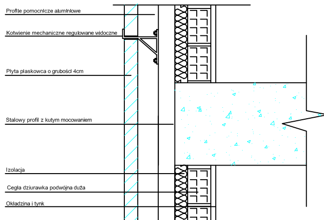
KONSTRUKCJA POMOCNICZA MIĘDZY ELEMENTAMI KUTYMI Z WIDOCZNYM KOTWIENIEM
