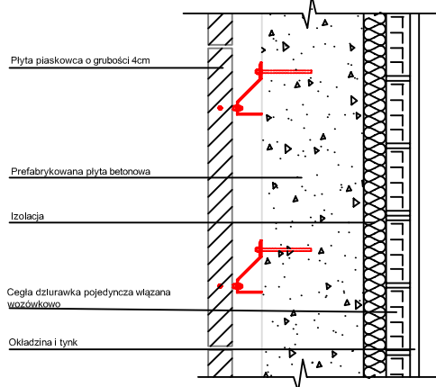
KOTWIENIE BEZPOŚREDNIE REGULOWANE BOCZNE DO PŁYTY BETONOWEJ
