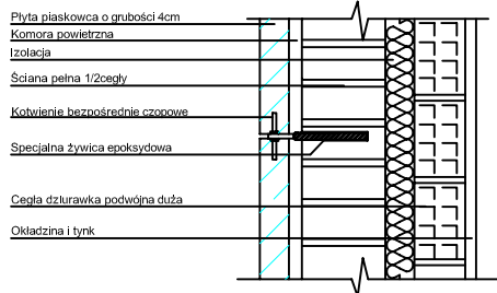
KOTWIENIE BEZPOŚREDNIE DO CEGŁY PEŁNEJ
