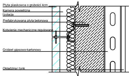
KOTWIENIE BEZPOŚREDNIE REGULOWANE DO PŁYTY BETONOWEJ
