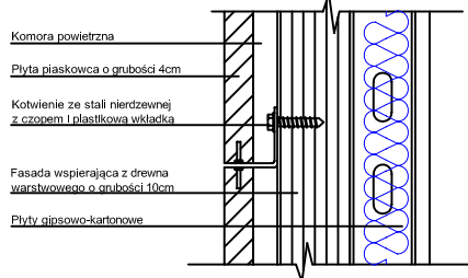
KOTWIENIE STAŁE BEZPOŚREDNIE DO DREWNA WARSTWOWEGO
