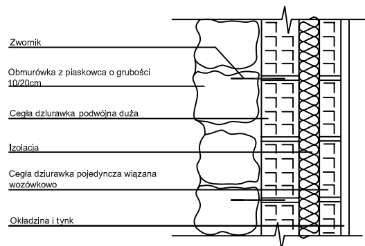
ŚCIANA NOŚNA Z OBMURÓWKĄ
