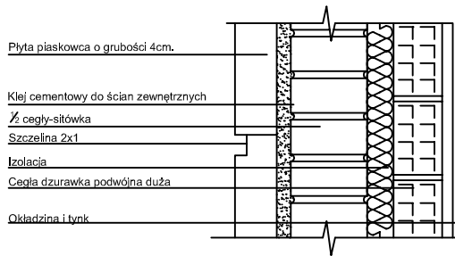
KLEJENIE DO PODWÓJNEJ DZIURAWKI
