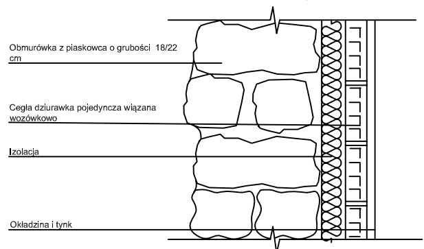
ŚCIANA NOŚNA Z DWUWARSTOWĄ OBMURÓWKĄ
