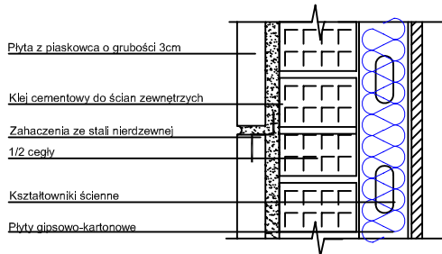
KLEJENIE DO PODWÓJNEJ DZIURAWKI
