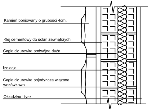
KAMIEŃ DŁUTOWANY KLEJONY DO PODWÓJNEJ DZIURAWKI
